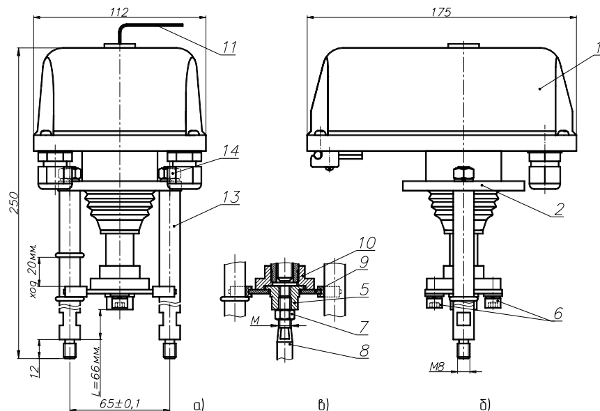
Рисунок 1. Электропривод ВЭП-115-1500
