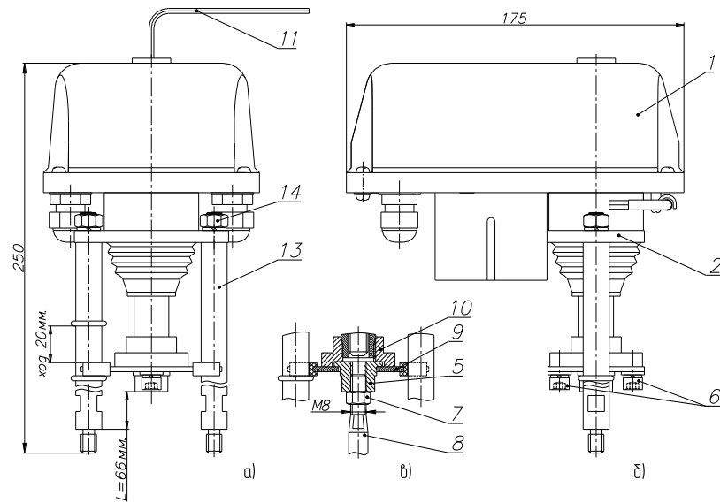
Рисунок 1. ВЭП-115-1500/40-20-220В
