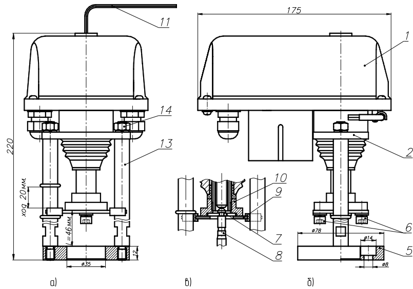
Рисунок 1. Электропривод ВЭП-118-3000
