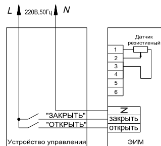
Рисунок 3. Схема подключения
