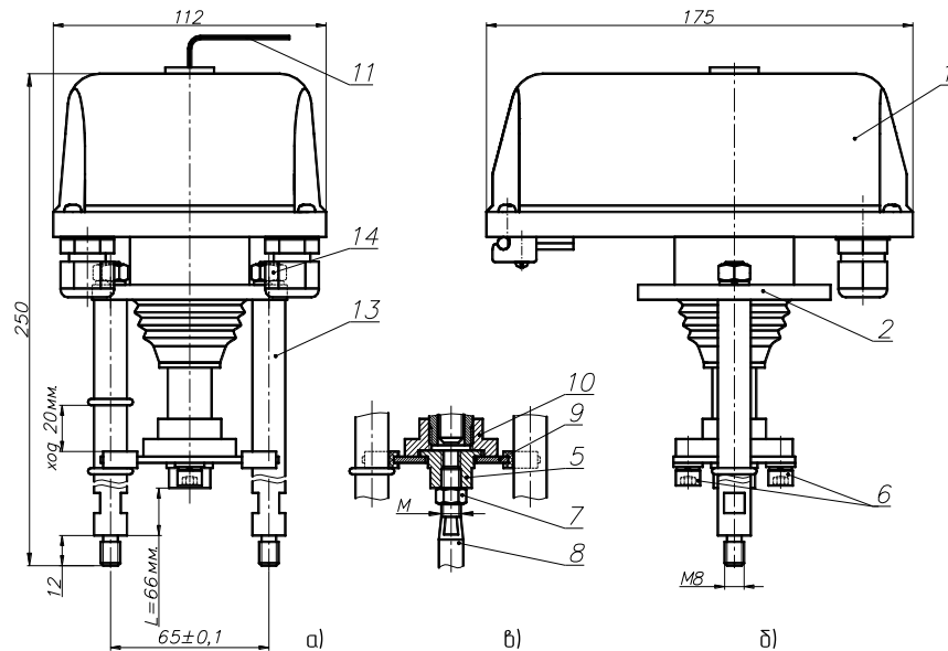
Рисунок 1. Электропривод ВЭП-115-1500/63-20-220В
