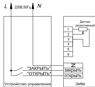
Рисунок 3. Схема подключения
