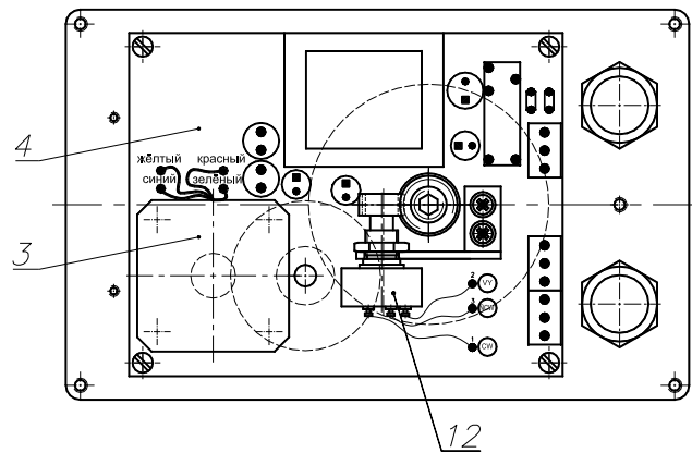
Рисунок 2. Электропривод (вид при снятой крышке)
