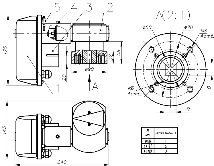
Рисунок 1. ВЭО-04-100/63-0,25-220В,50Гц
