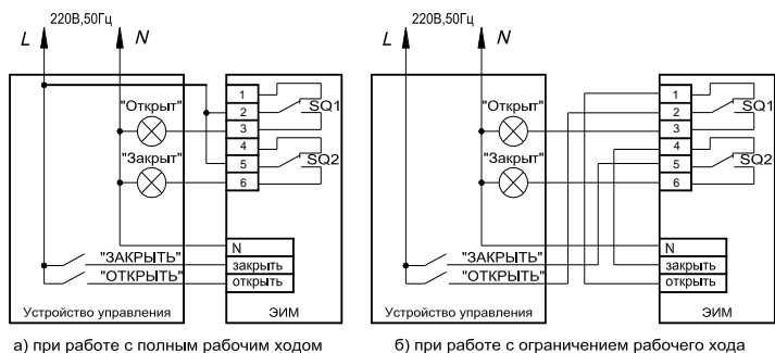
Рисунок 3. Схема подключения
