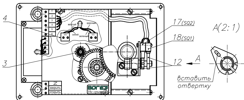
Рисунок 2. Электропривод ВЭМ-02 (вид при снятой крышке)
