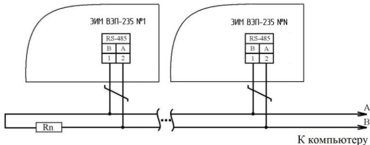
Рисунок 4.1 - Схема подключения ПК к ЭИМ ВЭП 235
