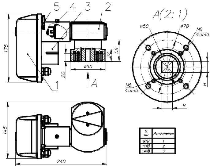
Рисунок 1. ВЭО-04-100/63-0,25-220В,50Гц
