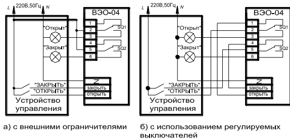
Рисунок 3. Схема подключения ВЭО-04
