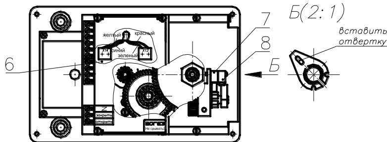
Рисунок 2. ВЭО-04 (вид при снятой крышке)
