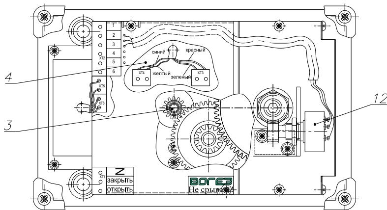
Рисунок 2. Электропривод (вид при снятой крышке)
