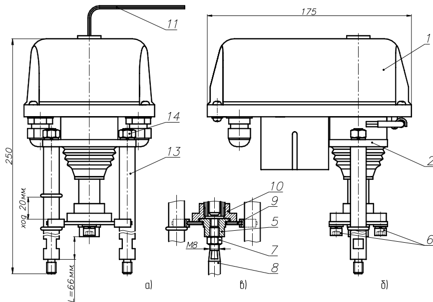
Рисунок 1 ВЭП-115-3000
