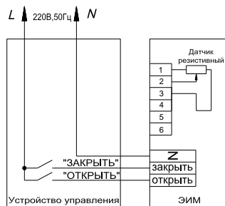
Рисунок 3. Схема подключения
