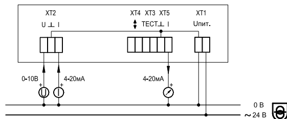
Рисунок 3. Схема подключения
