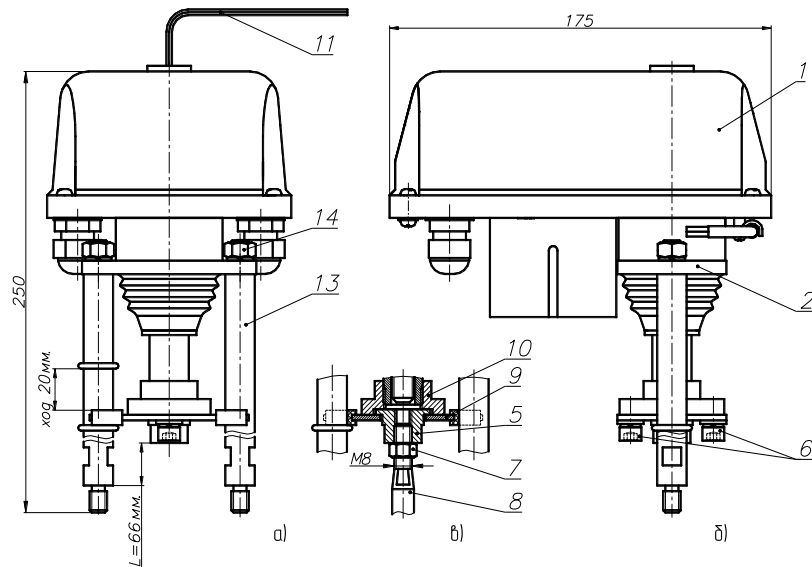
Рисунок 1. Электропривод ВЭП-115-1500
