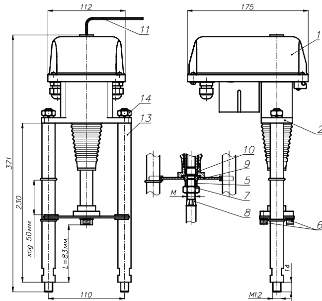
Рисунок 1. Электропривод ВЭП-115-4000
