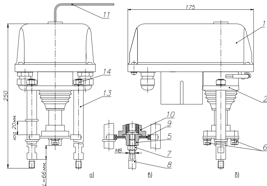
Рисунок 1. Электропривод ВЭП-115-3000
