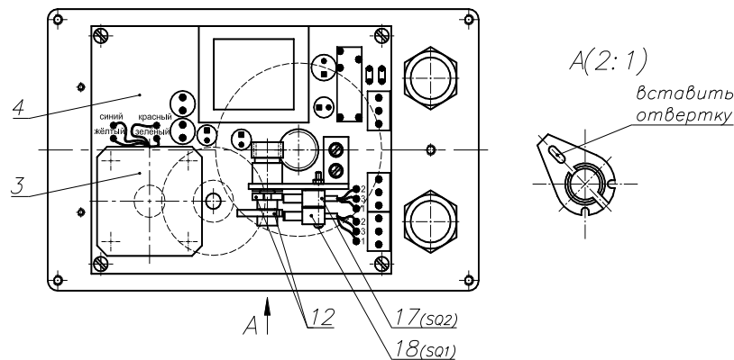
Рисунок 2 Электропривод (вид при снятой крышке)
