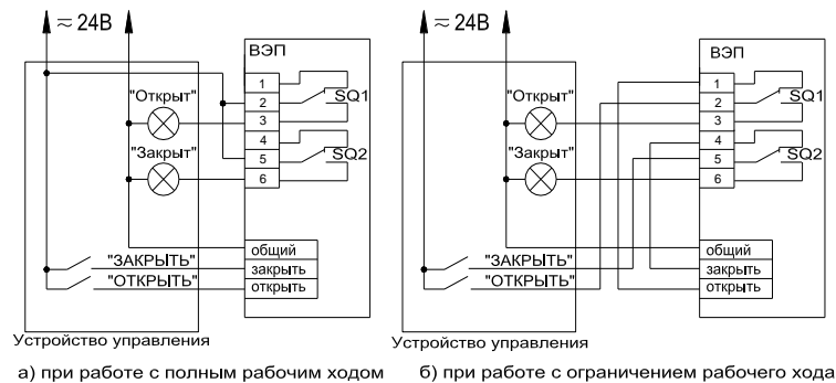
Рисунок 3. Схема подключения
