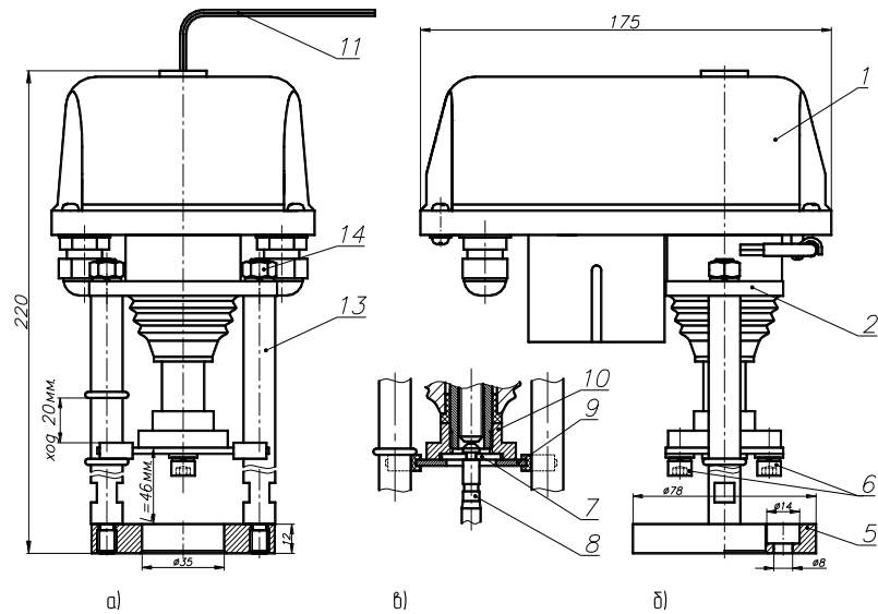
Рисунок 1. ВЭП-118-3000/63-20-220В
