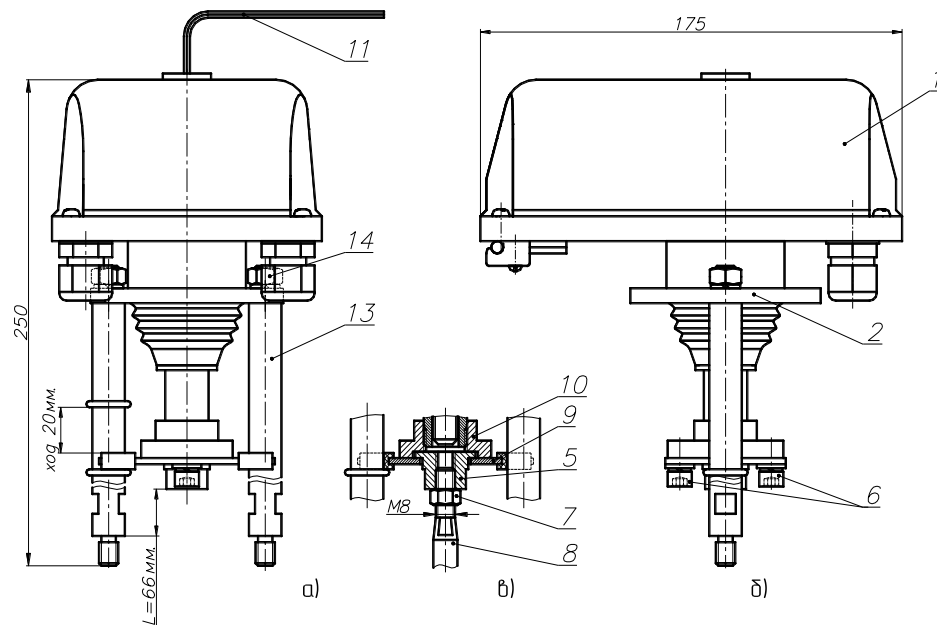
Рисунок 1. ВЭП-115-1500
