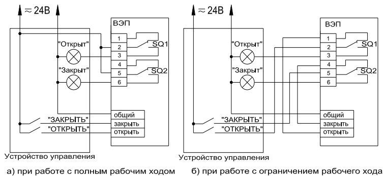
Рисунок 3. Схема подключения
