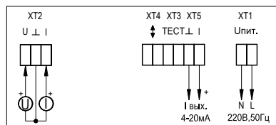
Рисунок 3. Схема подключения
