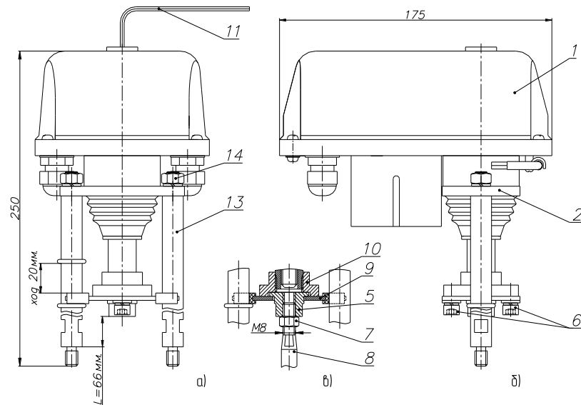
Рисунок 1. ВЭП-115-4000/63-20-220В
