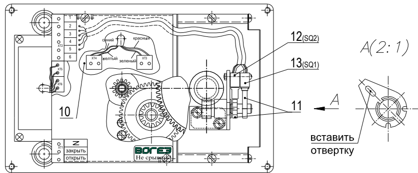
Рисунок 2. Электропривод (вид при снятой крышке),
