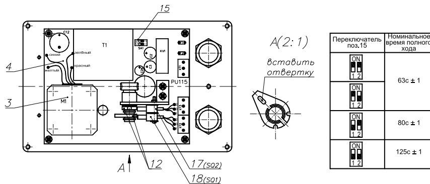
Рисунок 2 Электропривод (вид при снятой крышке)
