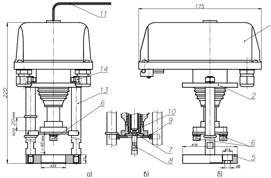
Рисунок 1. Электропривод ВЭП-118-1500
