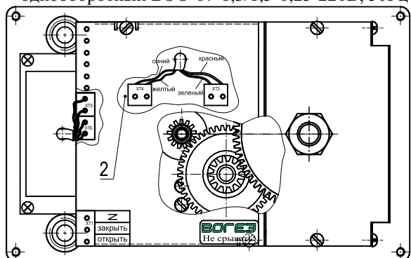
Рисунок 2. Электропривод (вид при снятой крышке),
