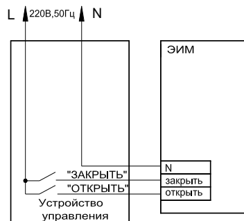
Рисунок 3. Схема подключения
