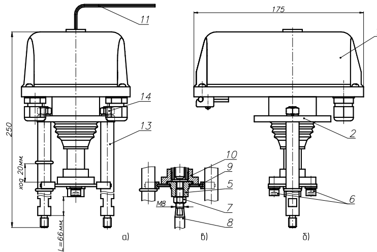
Рисунок 1. ВЭП-135-1500
