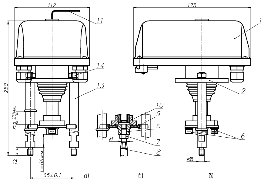
Рисунок 1 ВЭП-115-1500
