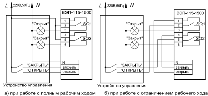
Рисунок 3 Схема подключения
