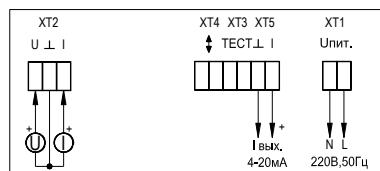
Рисунок 3. Схема подключения
