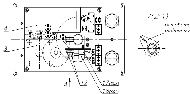
Рисунок 2. Электропривод (вид при снятой крышке)
