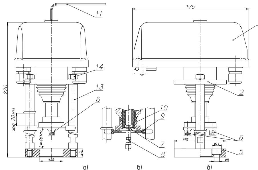
Рисунок 1. ВЭП-118-1500
