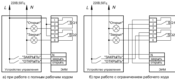
Рисунок 3. Схема подключения
