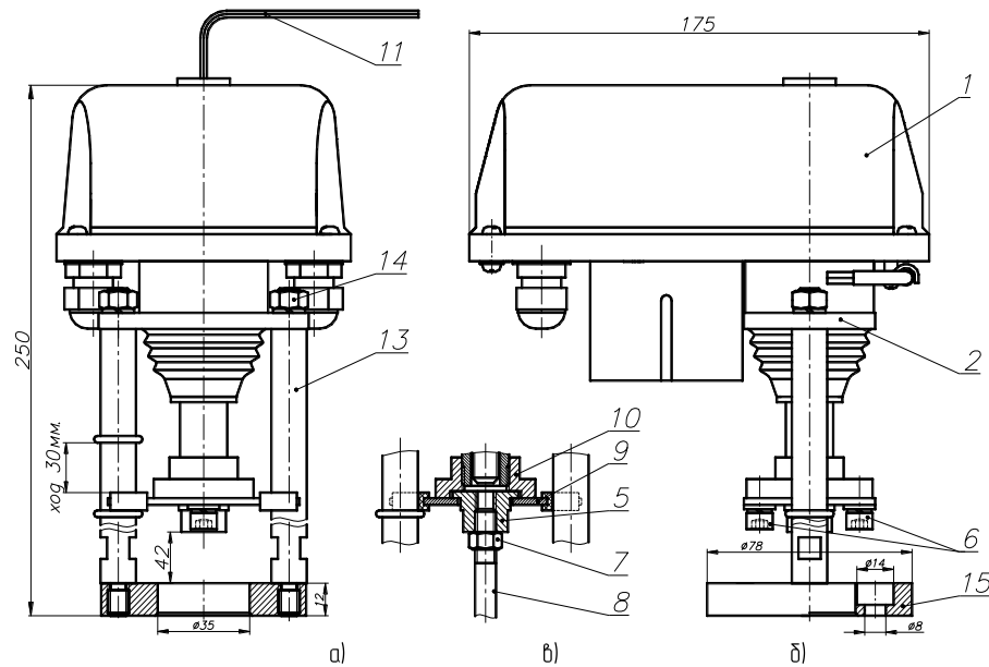
Рисунок 1. Электропривод ВЭП-118-3000
