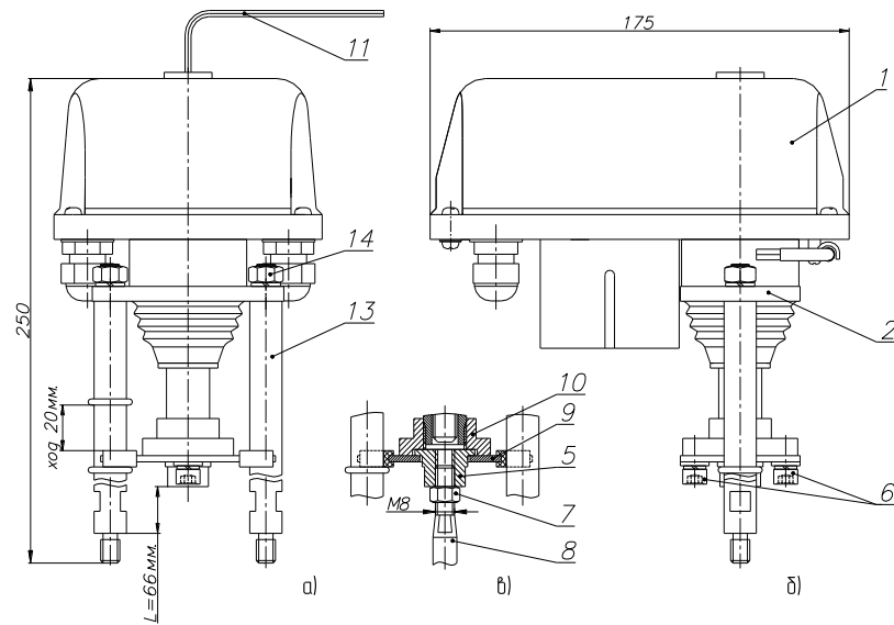
Рисунок 1. ВЭП-115-3000/63-20-220В
