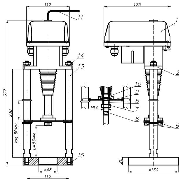
Рисунок 1. Электропривод ВЭП
