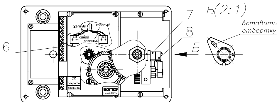
Рисунок 2 Электропривод (вид при снятой крышке)
