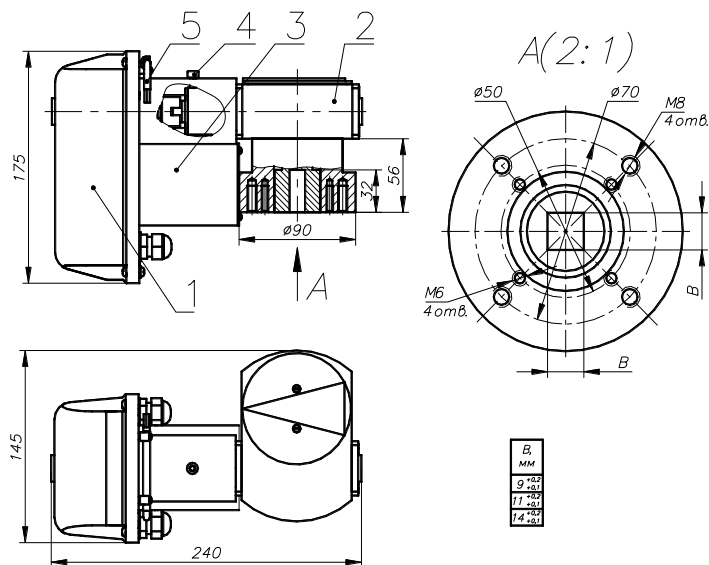
Рисунок 1 ВЭО-15-150/63-0,25-220В,50Гц
