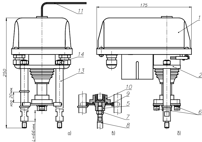
Рисунок 1. Электропривод ВЭП-115-3000
