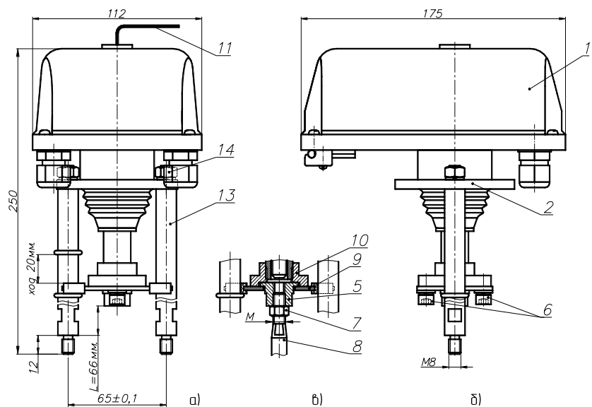
Рисунок 1. Электропривод ВЭП-115-1500
