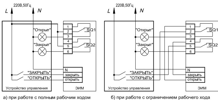
Рисунок 3. Схема подключения
