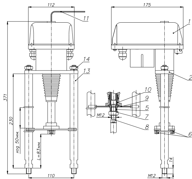
Рисунок 1. Электропривод ВЭП-115-4000
