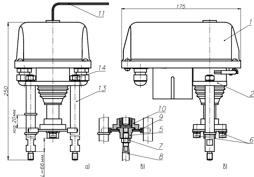
Рисунок 1. Электропривод ВЭП-115-3000
