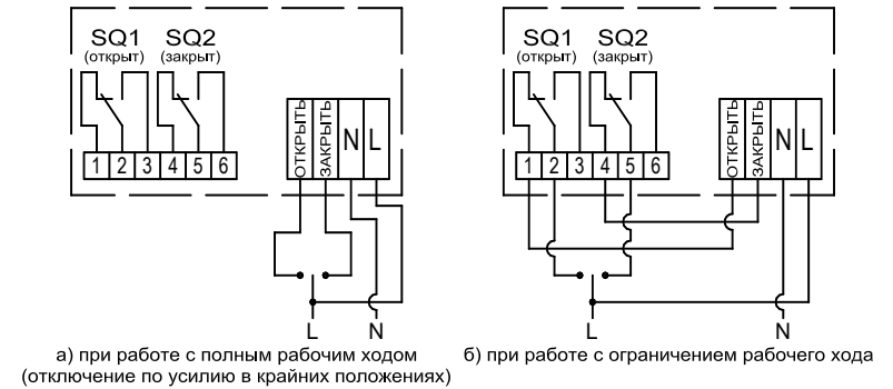
Рисунок 3 Схема подключения
