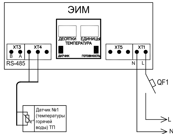
Рисунок 2 - Схема подключения ЭИМ
