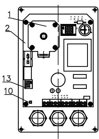
Рисунок 2. ВЭП-111МА-01 (вид при снятой крышке)
