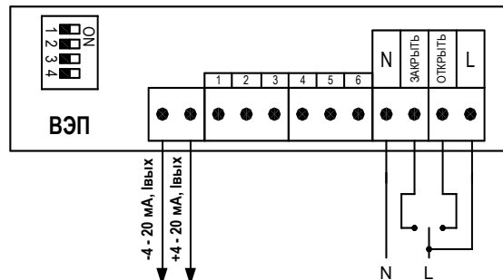
Рисунок - 3 Схема подключения
