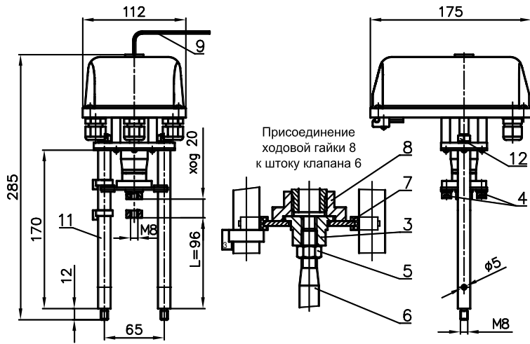
Рисунок 1. ВЭП-111МА-01
