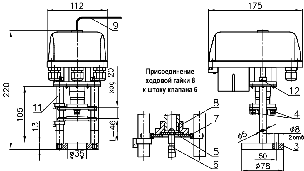
Рисунок 1. ВЭП-138МВ
