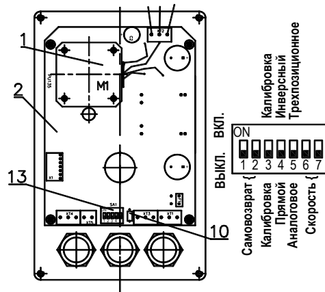
Рисунок 2. ВЭП-138МВ (вид при снятой крышке)
