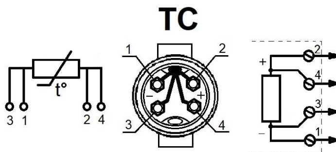
Рисунок В.3 Схема электрическая подключений ТС по четырехпроводной схеме
