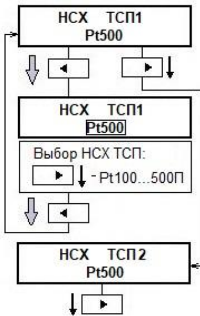
Рисунок Н.10 - Мнемосхема изменения параметра «НСХ ТСП»
