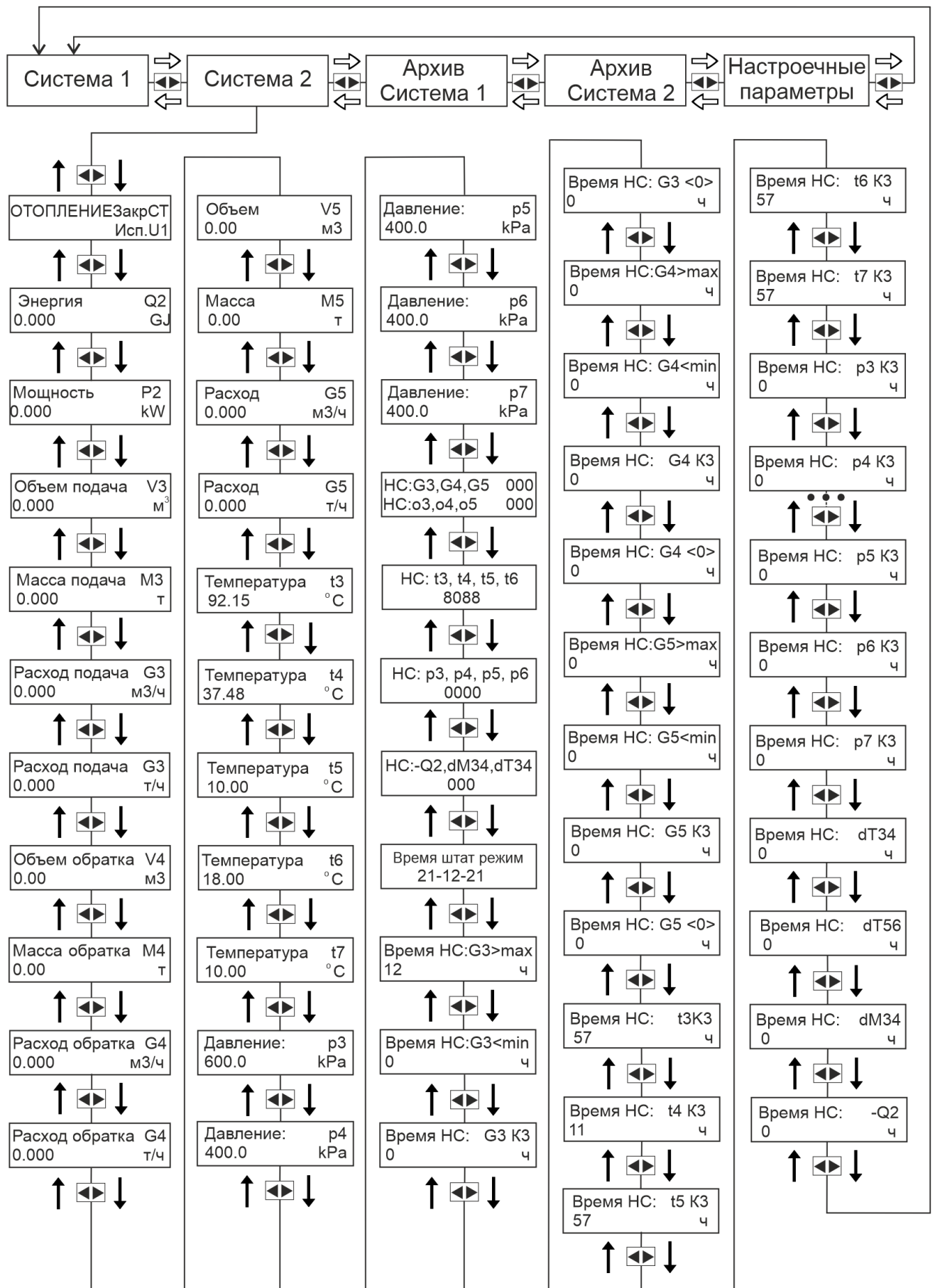
Рисунок И.2 – Схема перемещения по меню уровня СИСТЕМА 2
