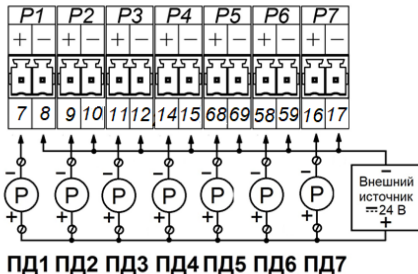
Рисунок В.2 Схема электрическая подключений ПД, питающихся от внешнего источника
