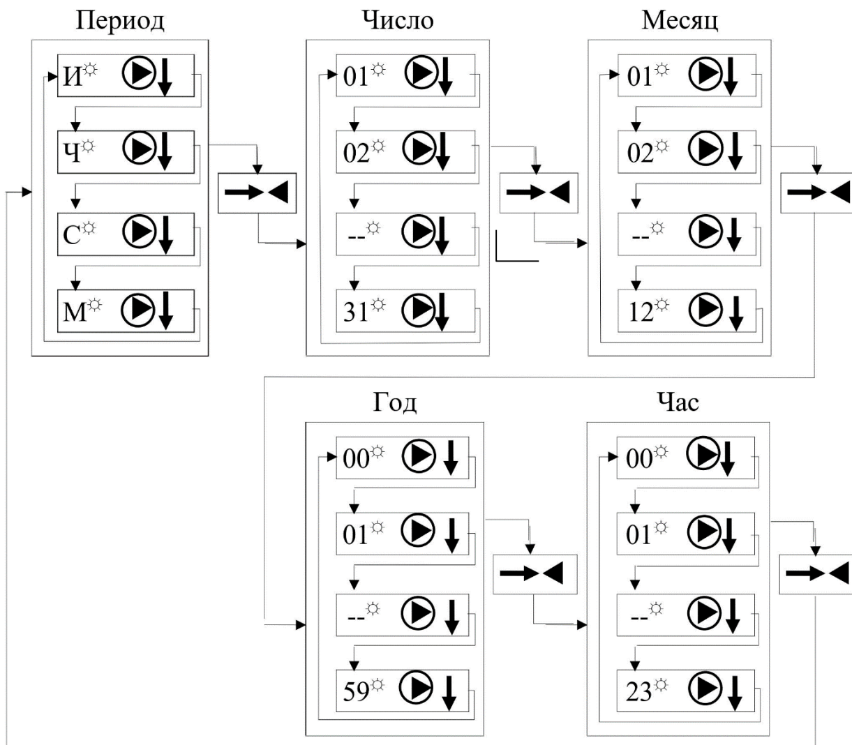
Рисунок 3 – Мнемосхема выбора периода, даты и времени архива
