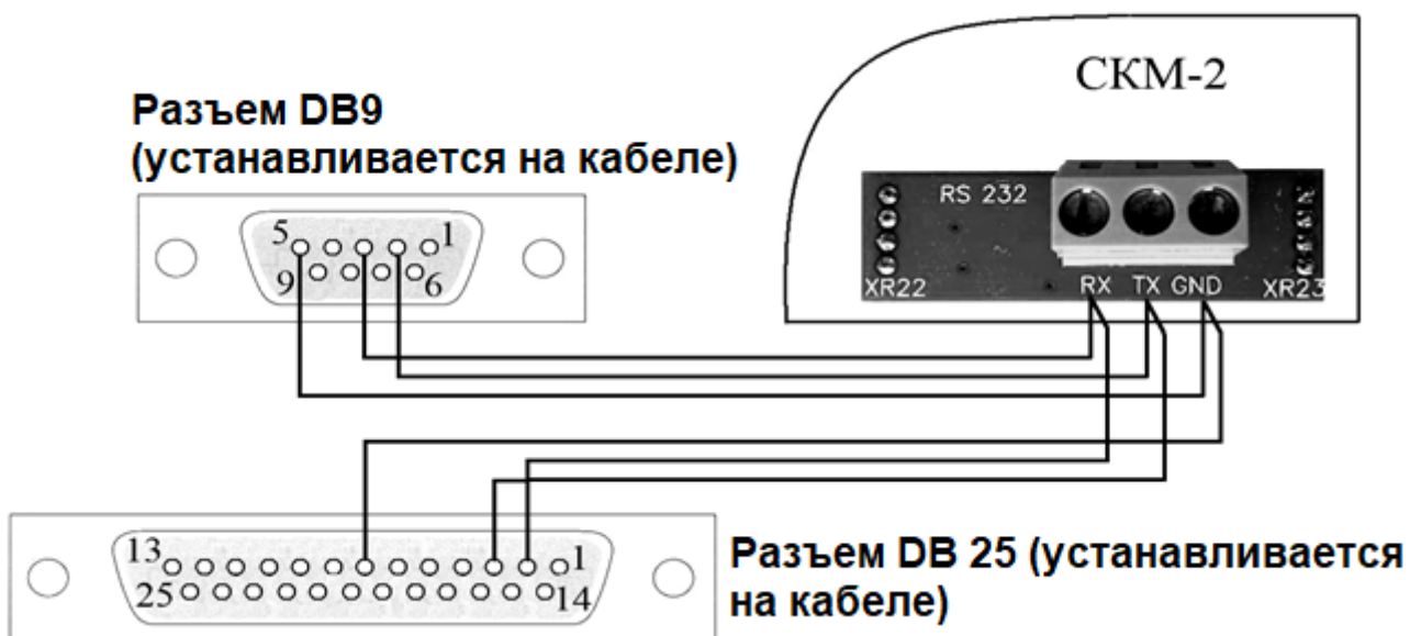
Рисунок В.6 – Схема подключения счетчика к модему
