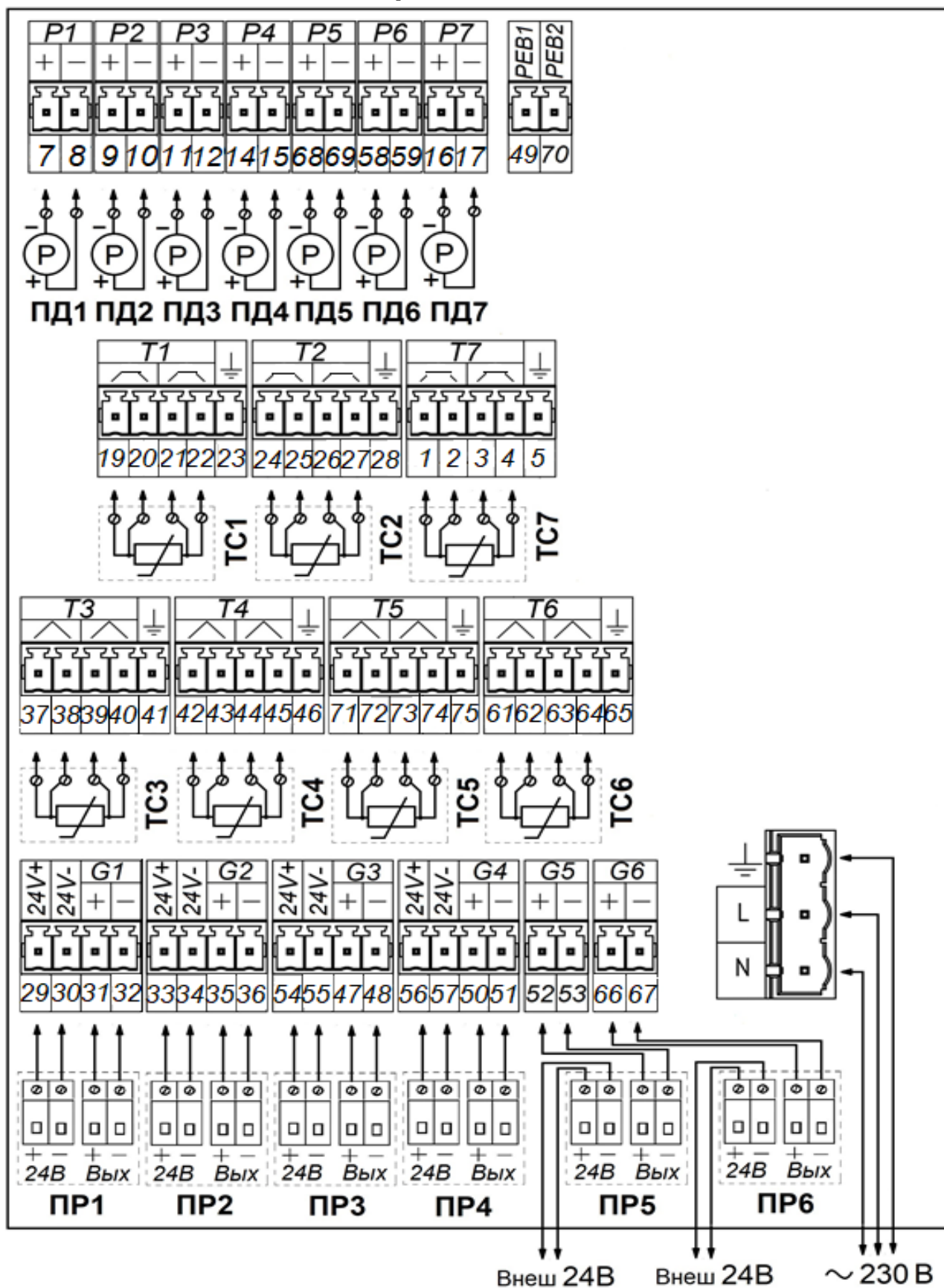
Рисунок В.1 Схема электрическая подключений.
