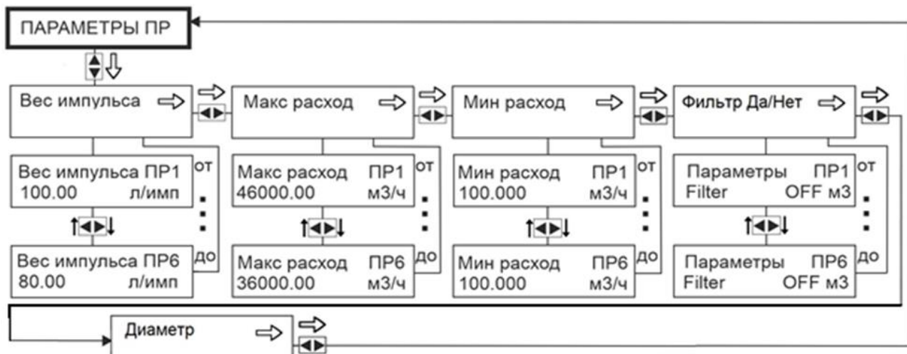
Рисунок М.1 – Схема перемещения по подменю ПАРАМЕТРЫ ПР
