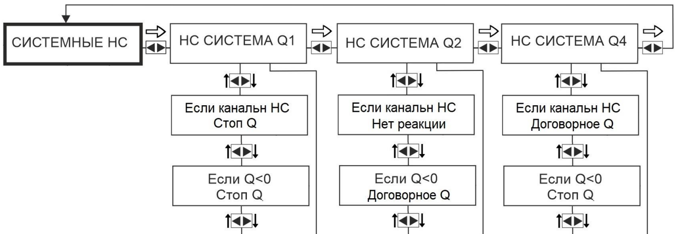
Рисунок М.6 – Схема перемещения по подменю СИСТЕМНЫЕ НС
