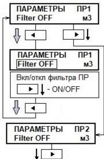
Рисунок Н.7 - Мнемосхема изменения параметра «Фильтр Да/Нет»
