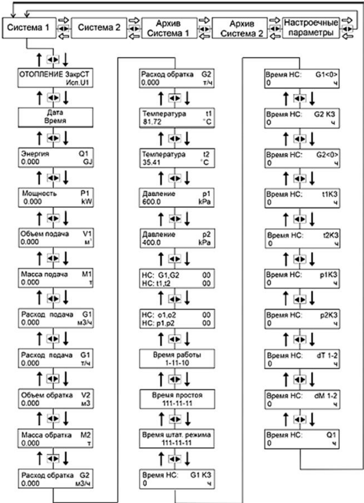
Рисунок И.1 – Схема перемещения по меню уровня СИСТЕМА 1
