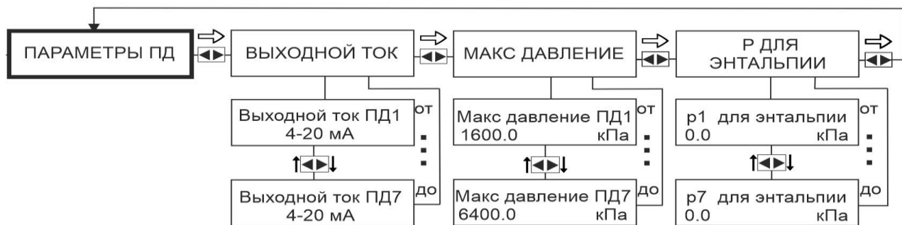
Рисунок М.3 – Схема перемещения по подменю ПАРАМЕТРЫ ПД
