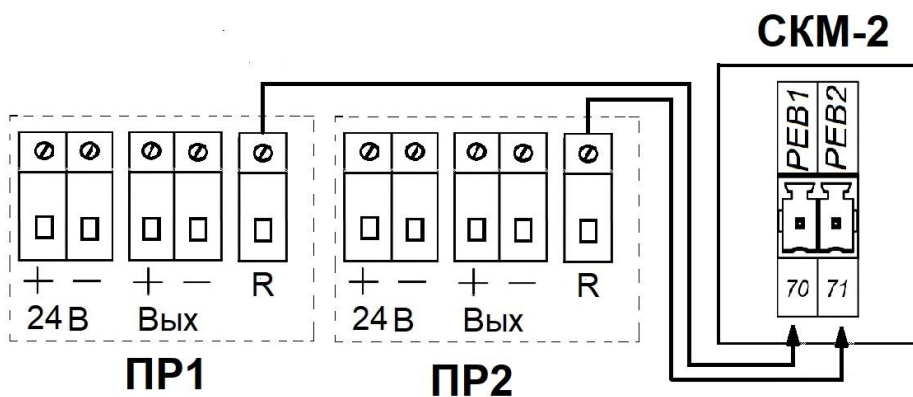
Рисунок В.3 Схема электрическая подключений ТС по четырехпроводной схеме
