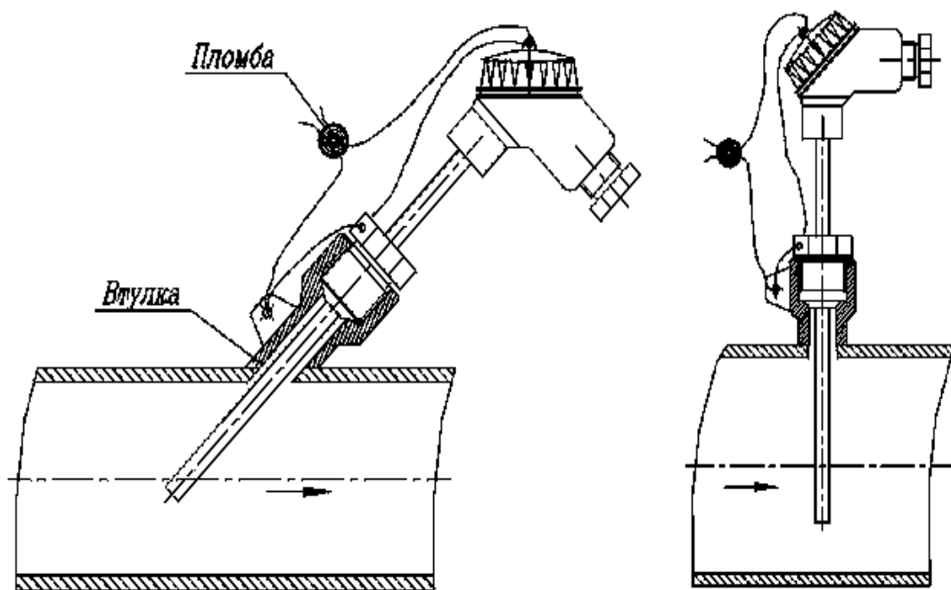
а) для трубопровода DN \leq 50 б) для трубопровода DN > 50
