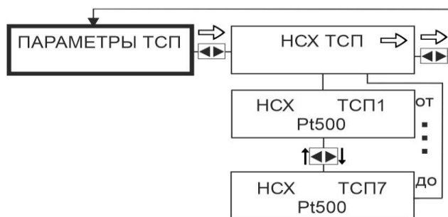
Рисунок М.2 – Схема перемещения по подменю ПАРАМЕТРЫ ТСП
