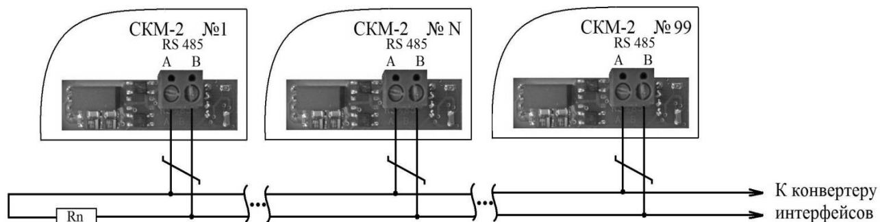
Рисунок В.7 – Схема организации сети на базе интерфейса RS-485
