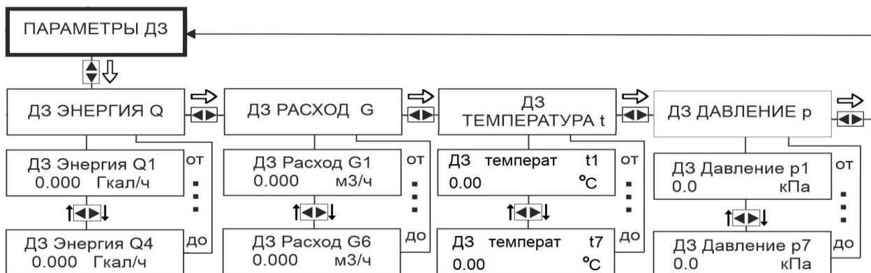
Рисунок М.4 – Схема перемещения по подменю ПАРАМЕТРЫ Д3
