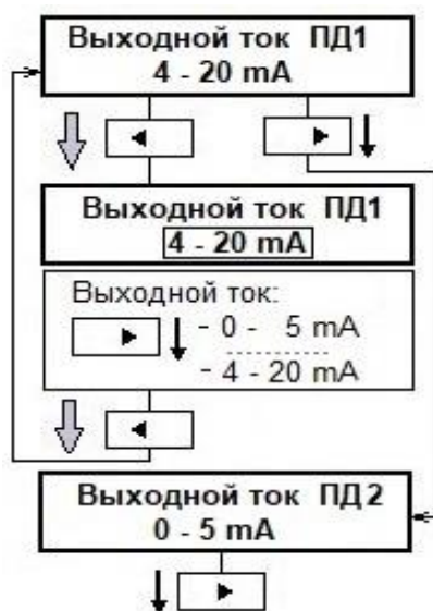
Рисунок Н.9 - Мнемосхема изменения параметра «Выходной ток»
