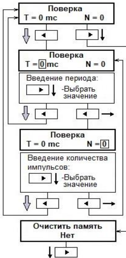
Рисунок Н.14 - Мнемосхема изменения параметра «Поверка»
