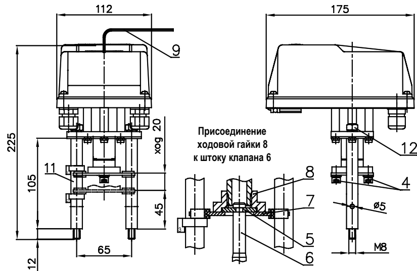
Рисунок 1. ВЭП-115МА-К
