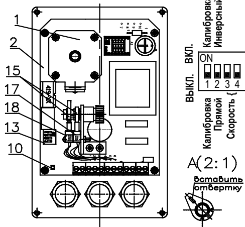
Рисунок 2. ВЭП-115МА-К (вид при снятой крышке)
