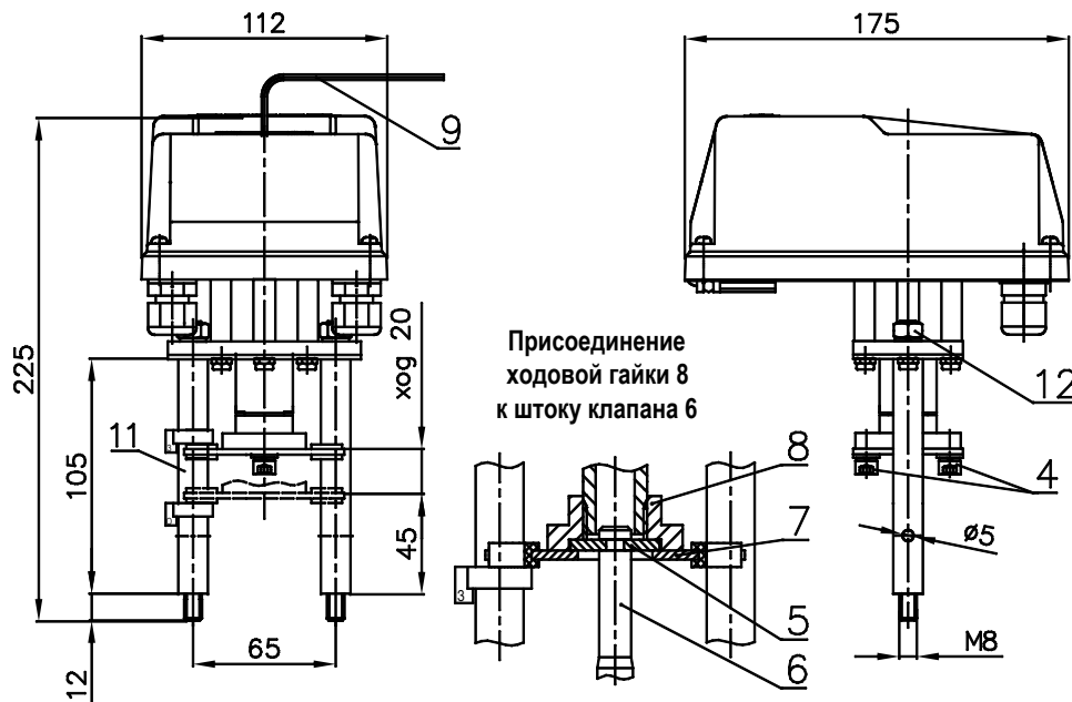
Рисунок 1 - ВЭП-115В-01-К
