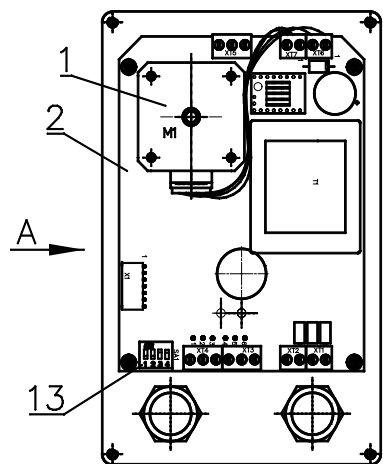
Рисунок 1 - ВЭП-115В-01-К
