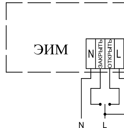
Рисунок 3 - Схема подключения
