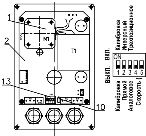
Рисунок 2. ВЭП-135М-К (вид при снятой крышке)
