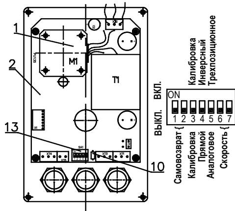
Рисунок 2. ВЭП-135МВ-К (вид при снятой крышке)
