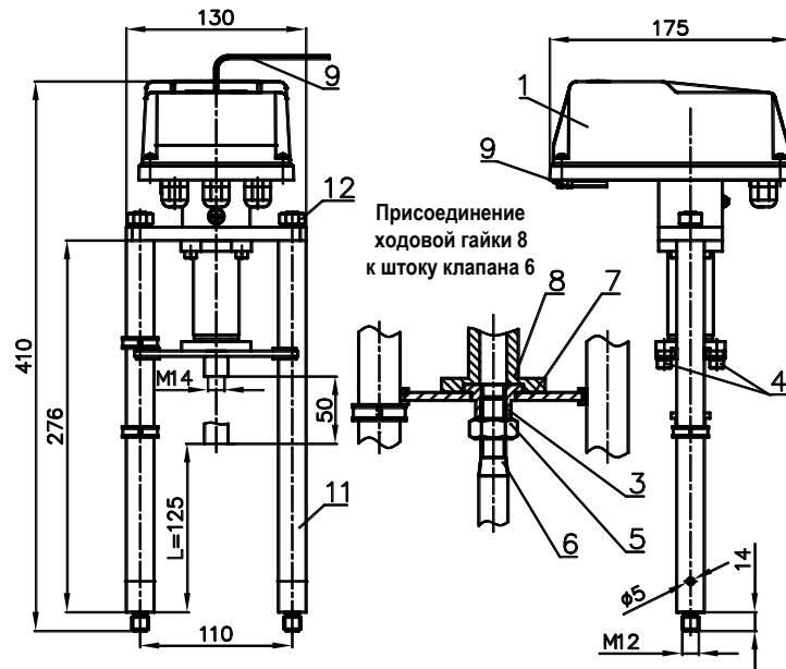
Рисунок 1 - ВЭП-135М
