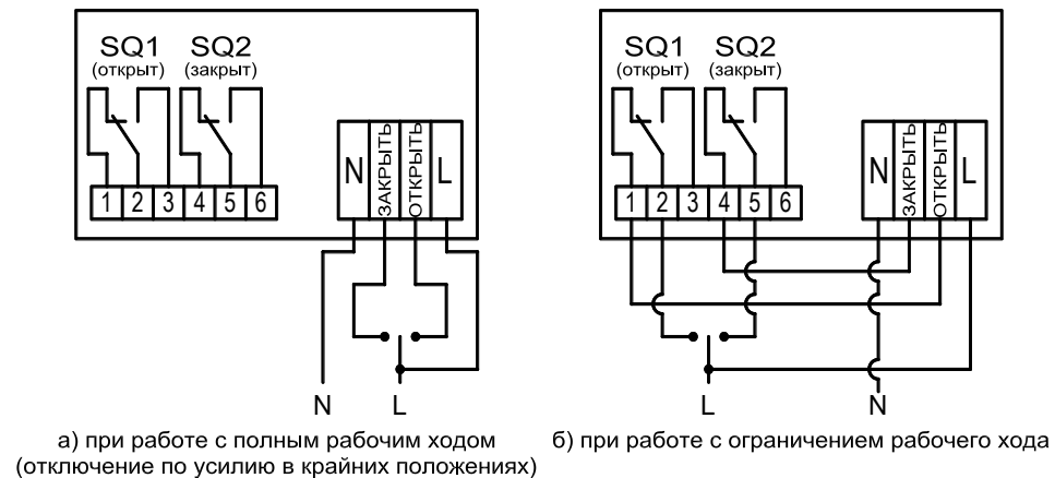
Рисунок 3 - Схема подключения
