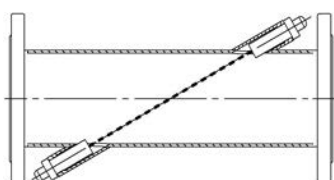
Прямая труба с однолучевым зондированием
