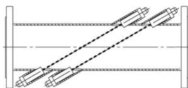
Прямая труба с многолучевым зондированием
