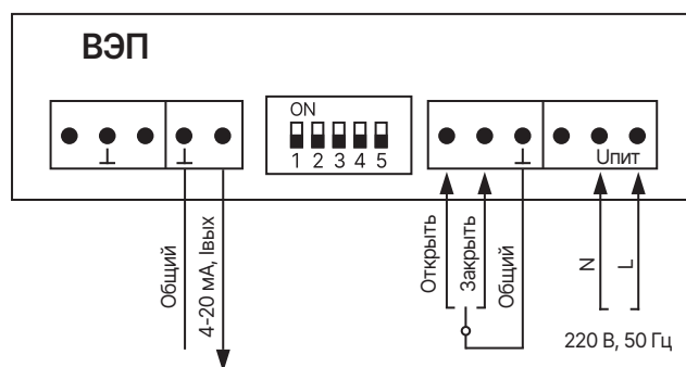
б) Схема подключения с управлением трехпозиционным сигналом (беспотенциальный контакт или открытый коллектор)
