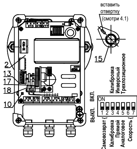
Рисунок 2. ВЭП-555В (вид при снятой крышке)
