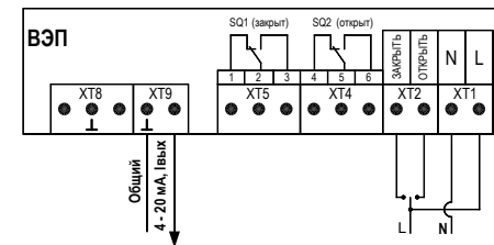
Рисунок 3.1 Схема подключения с управлением трехпозиционным сигналом при работе с полным рабочим ходом (220 В, 50 Гц).
