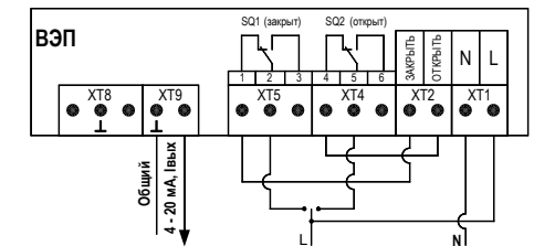
Рисунок 3.2 Схема подключения с управлением трехпозиционным сигналом при работе с ограничением рабочего хода (220 В, 50 Гц).
