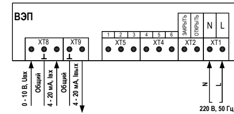
Рисунок 4. Схема подключения с управлением аналоговым сигналом.
