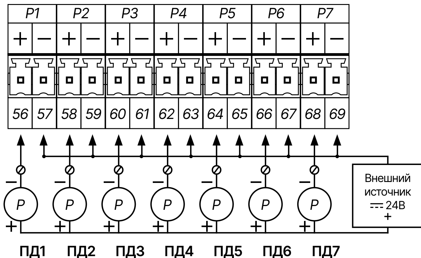
Схема электрических подключений ПД при питании от внешнего источника
