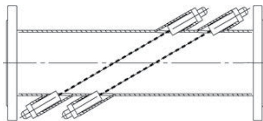
Прямая труба с многолучевым зондированием
