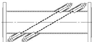
Прямая труба с многолучевым зондированием
