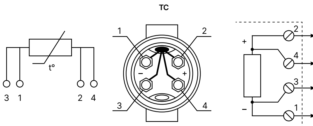
Схема электрических подключений ТС по четырехпроводной схеме
