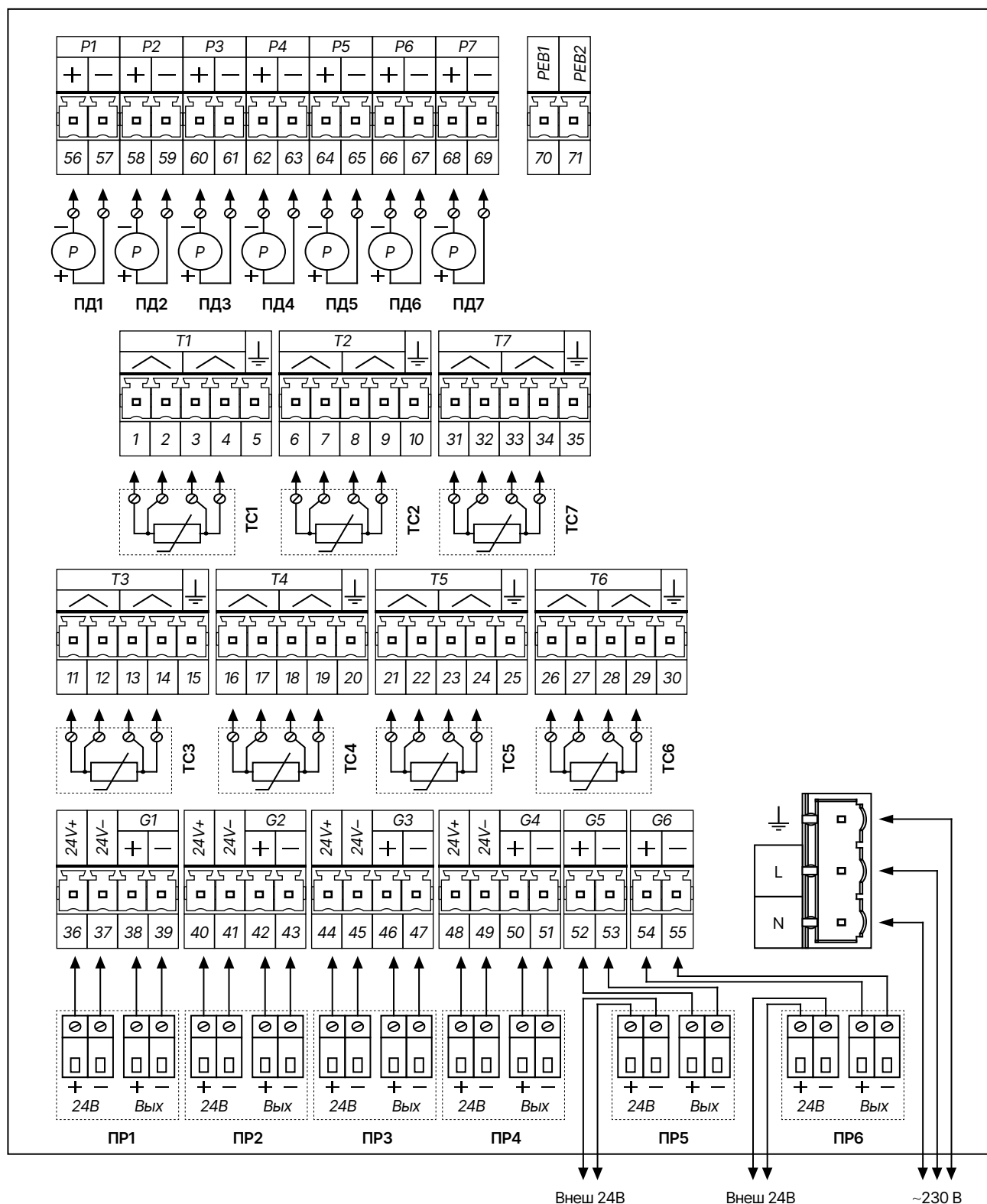
Схема электрических подключений
