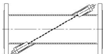
Прямая труба с однолучевым зондированием
