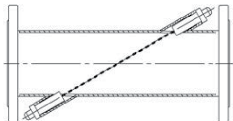
Прямая труба с однолучевым зондированием
